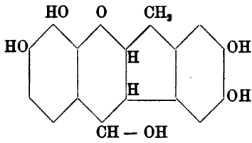
Hämatoxylin
